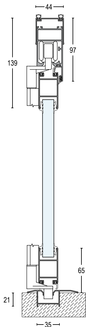
Guía empotrada
