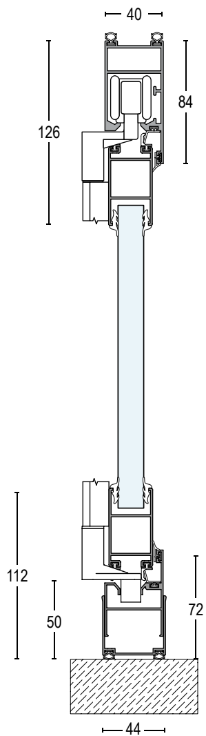
Guía superpuesta
